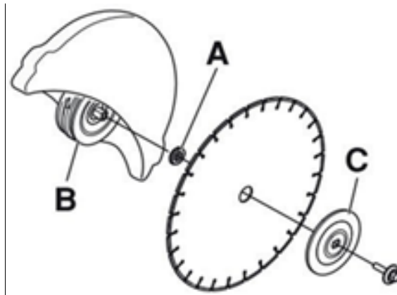
Рис.2 Установка диска
