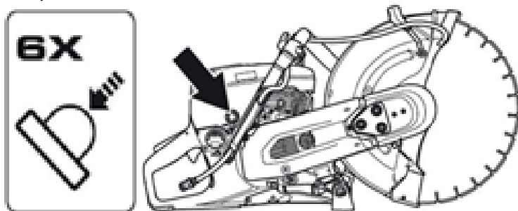
Рис. 9. Подкачка топлива праймером
